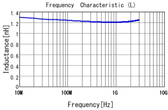
■ LQG15HN1N2B02 L
