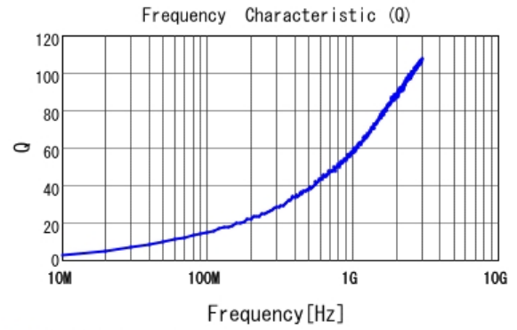
■ LQG15HN1N2B02 Q
