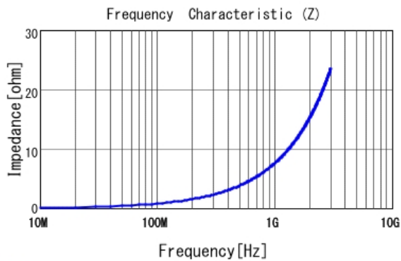
■ LQG15HN1N2B02 |Z|
