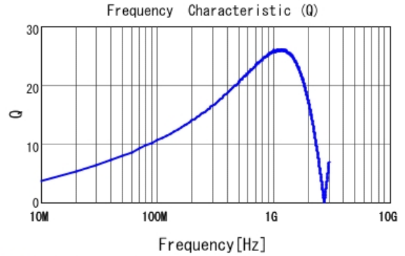
■ LQG15HN18NH02 Q
