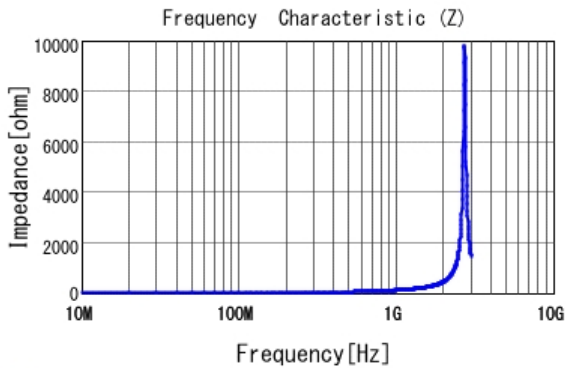
■ LQG15HN18NH02 |Z|
