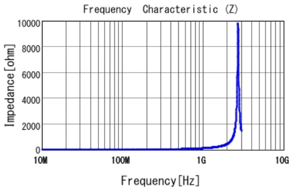
■ LQG15HN18NG02 |Z|
