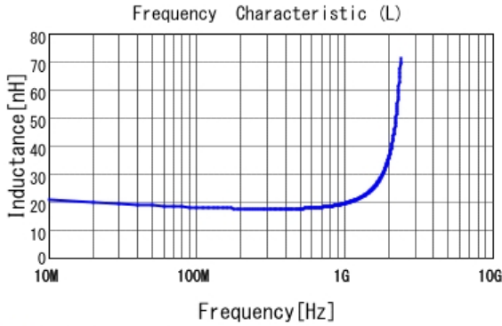
■ LQG15HN18NG02 L
