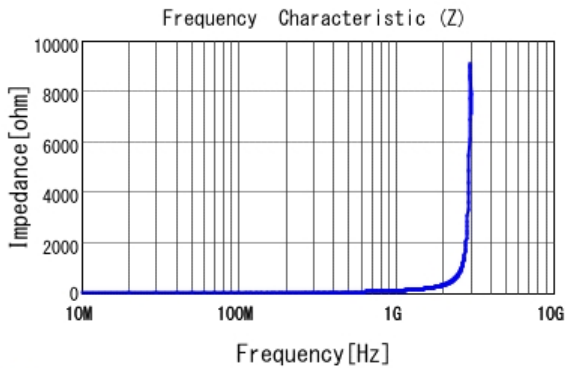
■ LQG15HN15NH02 |Z|
