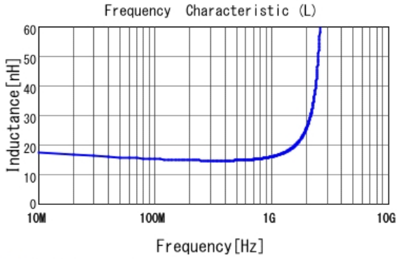
■ LQG15HN15NH02 L
