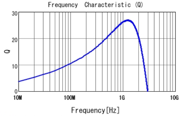
■ LQG15HN15NH02 Q
