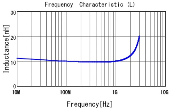
■ LQG15HN10NG02 L
