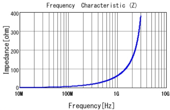
■ LQG15HN10NG02 |Z|
