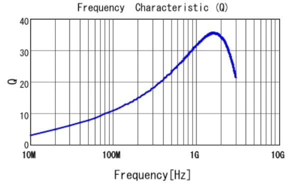
■ LQG15HN10NG02 Q
