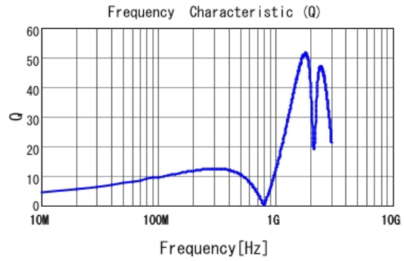
■ LQG15HHR12G02 Q
