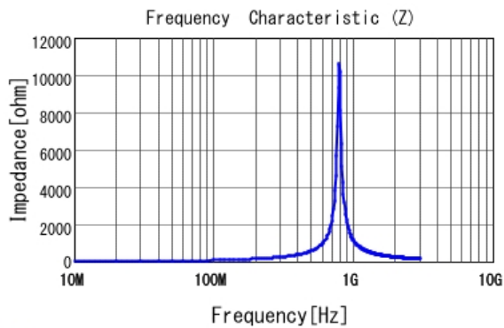
■ LQG15HHR12G02 |Z|
