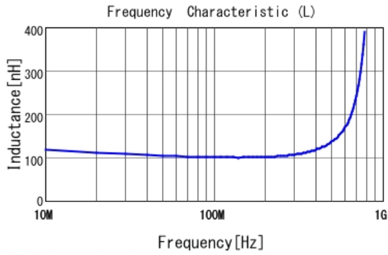
■ LQG15HHR10J02 L
