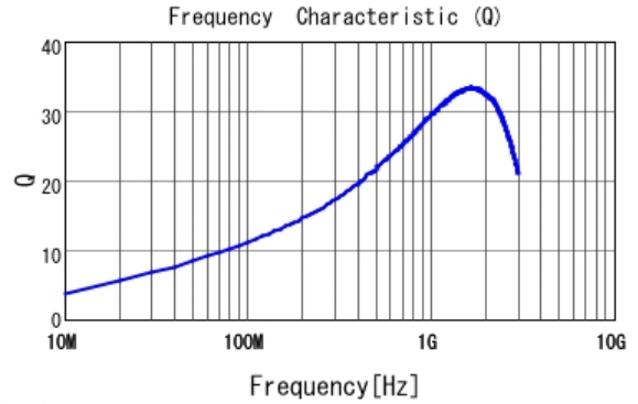
■ LQG15HH8N2J02 Q
