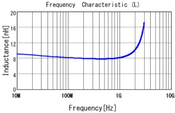
■ LQG15HH8N2J02 L
