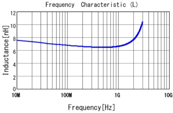
■ LQG15HH6N8J02 L
