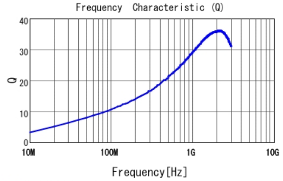
■ LQG15HH6N8J02 Q
