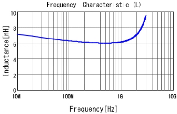
■ LQG15HH6N2B02 L
