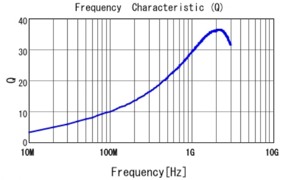
■ LQG15HH6N2B02 Q
