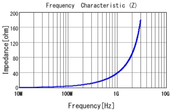
■ LQG15HH6N2B02 |Z|
