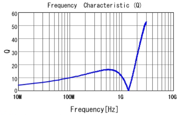
■ LQG15HH56NG02 Q
