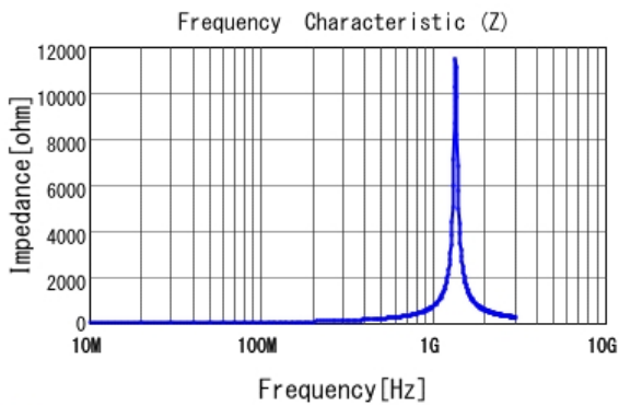
■ LQG15HH56NG02 |Z|
