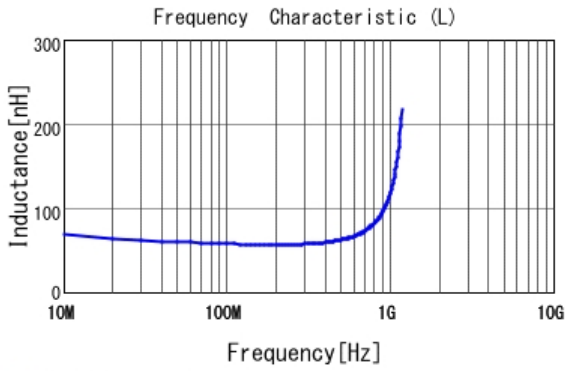
■ LQG15HH56NG02 L
