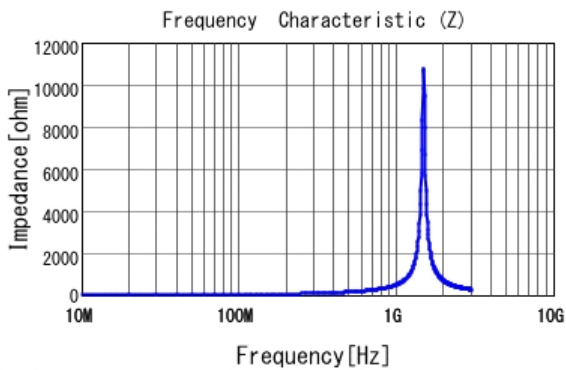
■ LQG15HH47NH02 |Z|
