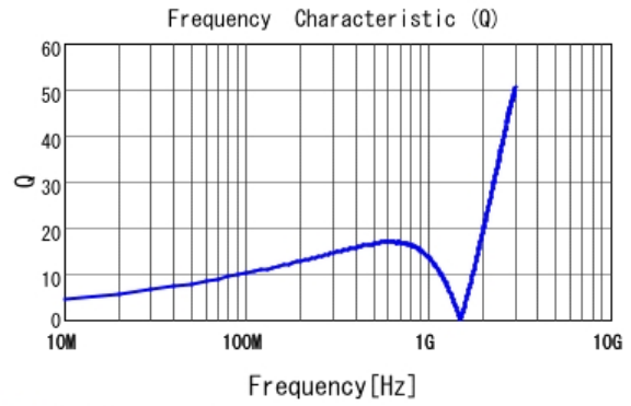
■ LQG15HH47NH02 Q
