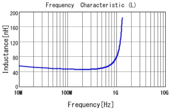
■ LQG15HH47NH02 L
