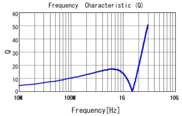
■ LQG15HH47NG02 Q
