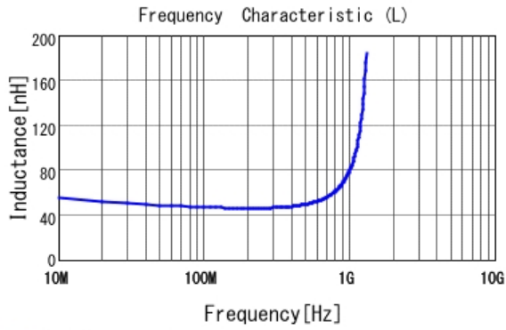
■ LQG15HH47NG02 L
