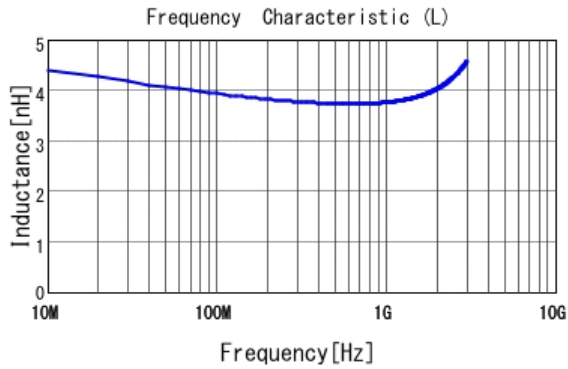
■ LQG15HH3N9S02 L
