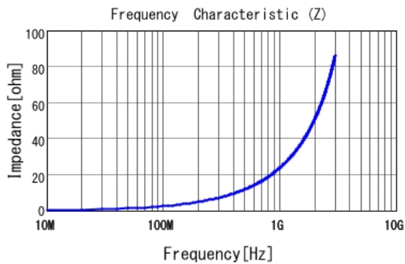
■ LQG15HH3N9S02 |Z|
