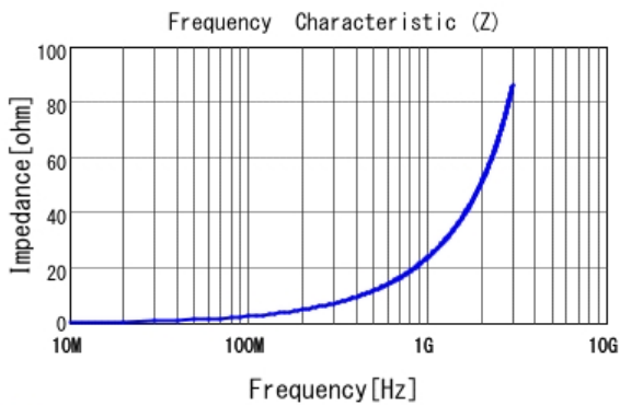
■ LQG15HH3N9B02 |Z|
