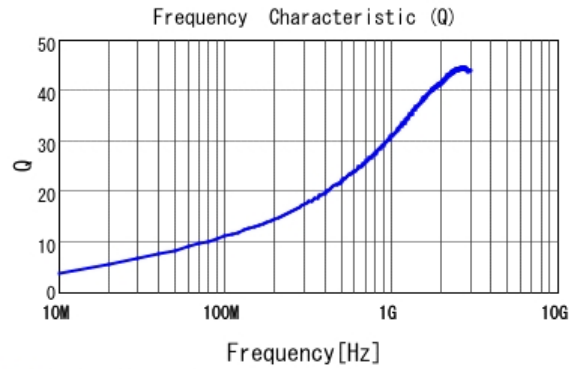
■ LQG15HH3N9B02 Q
