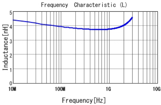
■ LQG15HH3N9B02 L
