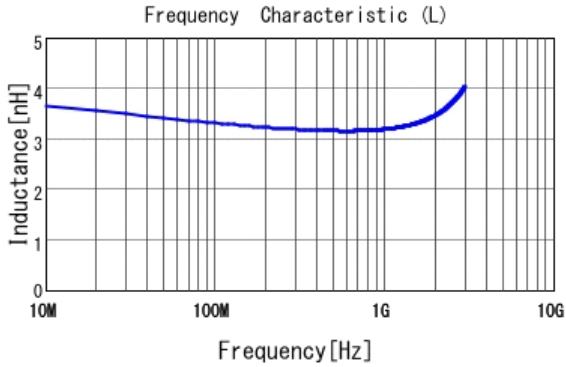
■ LQG15HH3N3B02 L
