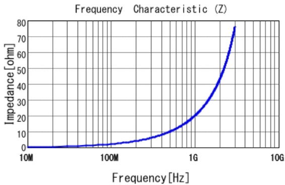
■ LQG15HH3N3B02 |Z|
