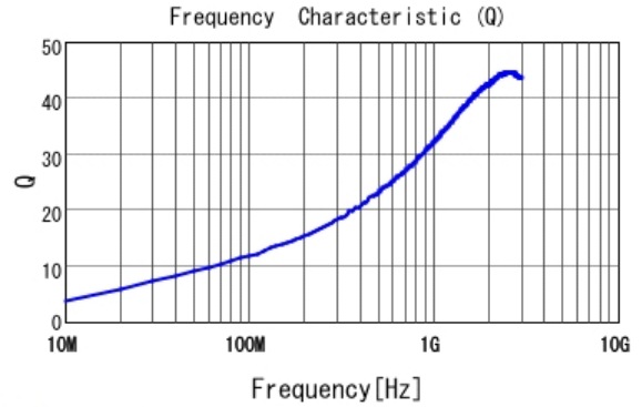
■ LQG15HH3N3B02 Q
