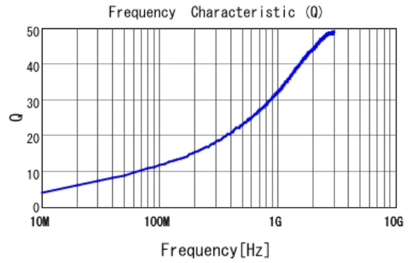
■ LQG15HH2N7B02 Q
