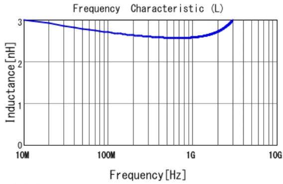
■ LQG15HH2N7B02 L
