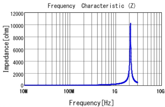
■ LQG15HH27NJ02 |Z|
