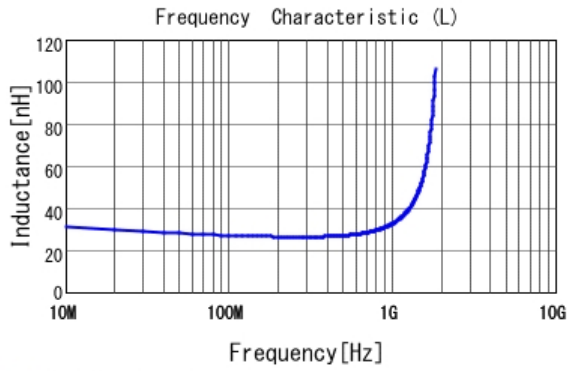
■ LQG15HH27NJ02 L
