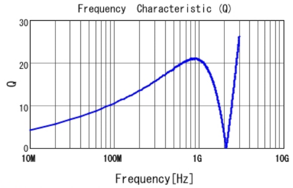
■ LQG15HH27NJ02 Q
