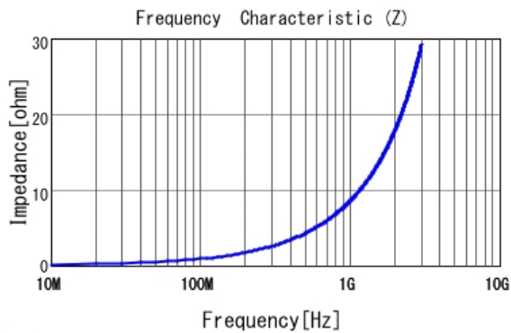
■ LQG15HH1N5S02 |Z|
