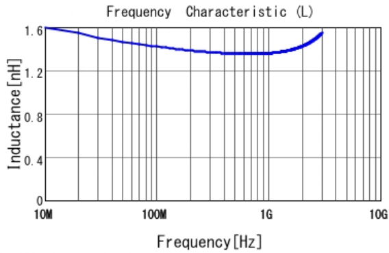
■ LQG15HH1N5S02 L
