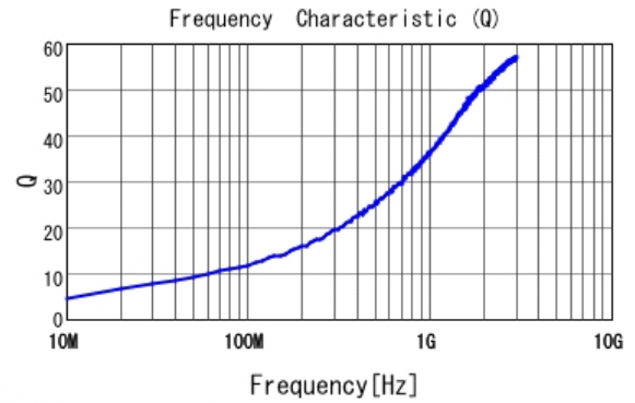
■ LQG15HH1N5S02 Q
