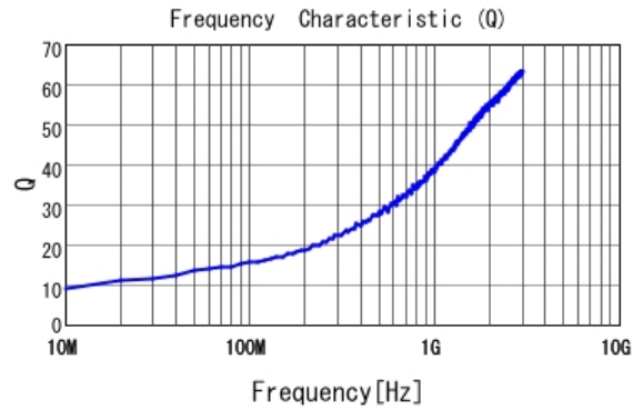
■ LQG15HH1N0B02 Q
