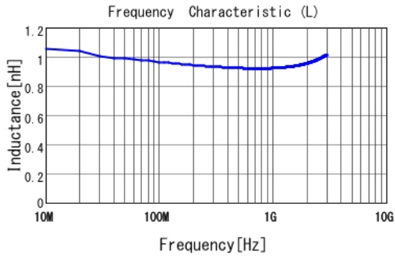
■ LQG15HH1N0B02 L
