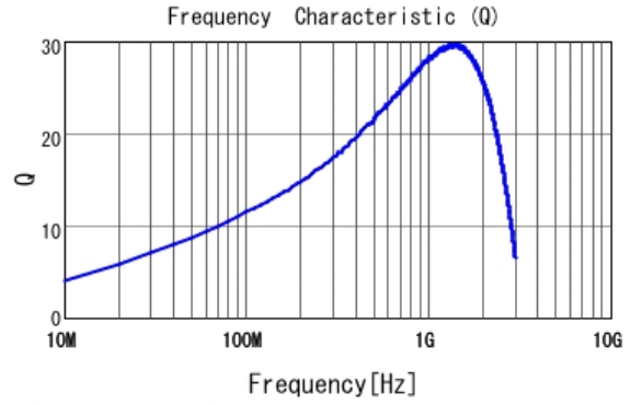
■ LQG15HH12NH02 Q
