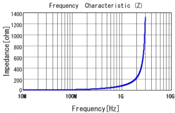
■ LQG15HH12NH02 |Z|
