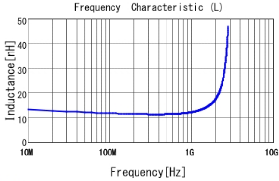
■ LQG15HH12NH02 L
