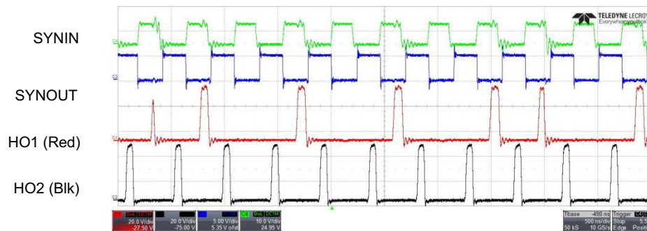
Figure 26. SYNIN (2.2 MHz) VIN 36 V
