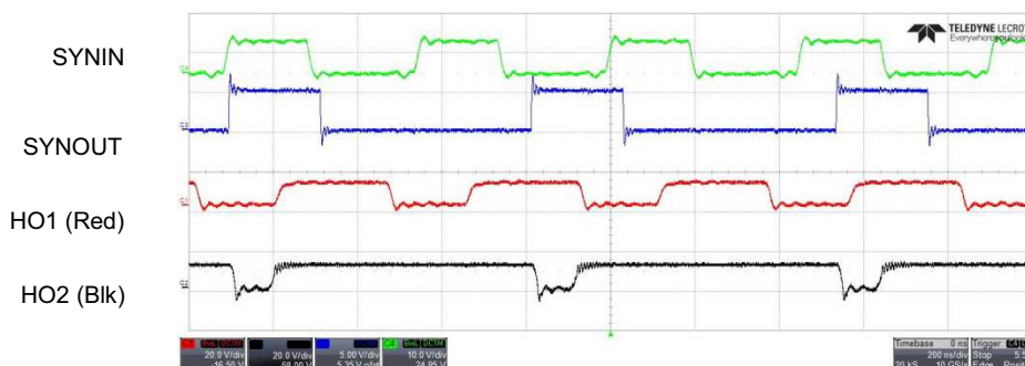
Figure 24. SYNIN (2.2 MHz) VIN 6.41 V
