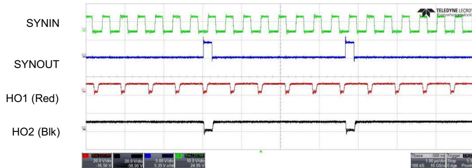
Figure 25. SYNIN (2.2 MHz) VIN 4.2 V
