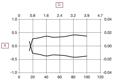
Fig. 4 Fast mode
