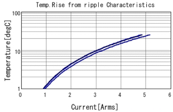
KRM55WR7YA476MH01 Temp. rise ■ 50kHz ■ 100kHz ■ 300kHz
