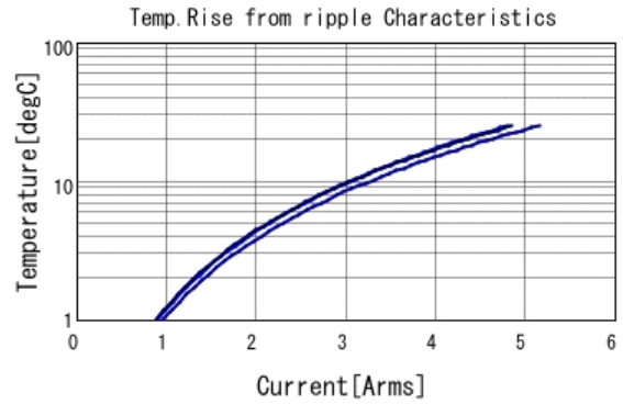
KRM55QR7YA226KH01 Temp. rise ■ 50kHz ■ 100kHz ■ 300kHz
