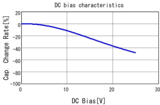
■ KCM55WR71E686MH01 C-DC bias capchange, 25.0degC, AC0.
