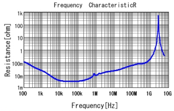
■ KCM55WR71E686MH01 R DCOV, 25degC
