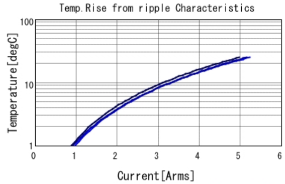
■ KCM55WR71E686MH01 Temp. rise ■ 50kHz ■ 100kHz ■ 300kHz
