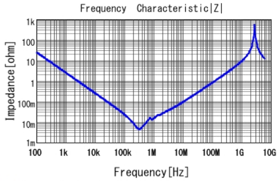
■ KCM55WR71E686MH01 |Z| DCOV, 25degC
