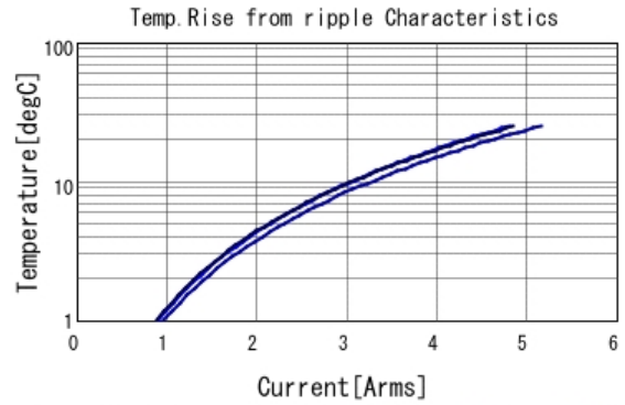
■ KCM55WR71E476MH01 Temp. rise ■ 50kHz ■ 100kHz ■ 300kHz
