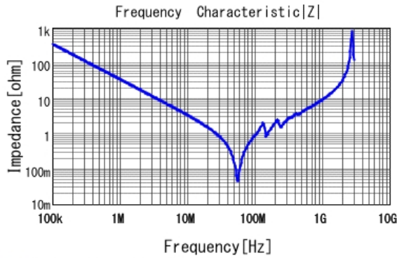
■ KCA55Q7UMF472KL01 |Z| DC0V, 25degC
