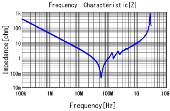
■ KCA55Q7UMF472KH01 |Z| DC0V, 25degC
