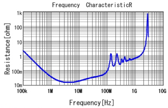
■ KCA55Q7UMF472KH01 R DC0V, 25degC
