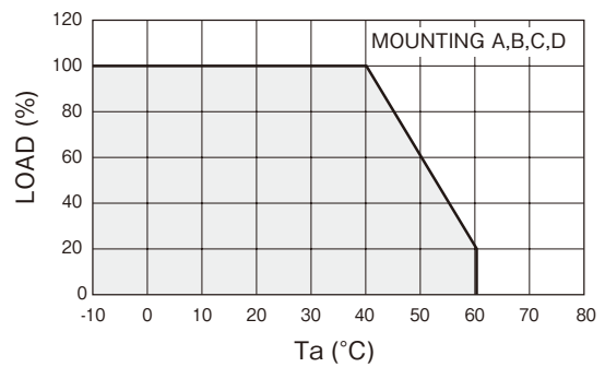
HWS30/A
