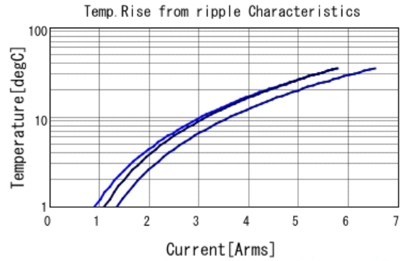
GRT32EC81C476KE13 Temp. rise ■ 60kHz ■ 300kHz ■ 600kHz
