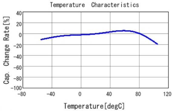
■ GRT32EC81C476KE13 C-Temp. capchange, DCO. 0V, ACO. 5Vrm
