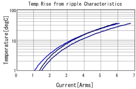
GRT32EC81A476KE13 Temp. rise ■ 60kHz ■ 300kHz ■ 600kHz
