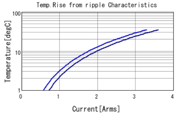
GRT155C71A225KE13 Temp. rise ■ 500kHz ■ 1MHz
