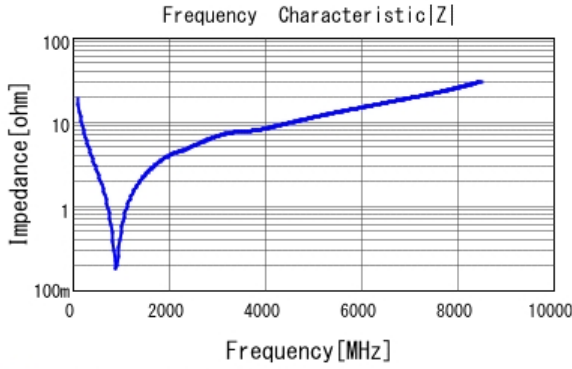
■ GRT1555C2A820JA02 |Z| DC0V, 25degC
