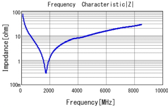
■ GRT1555C1E220JA02 |Z| DC0V, 25degC
