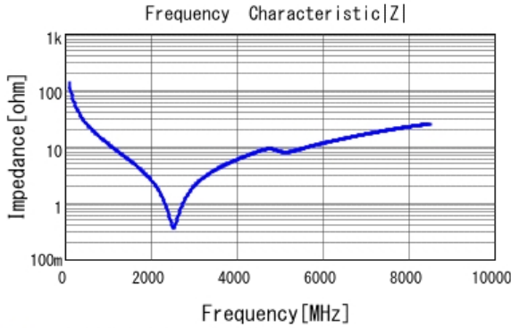
■ GRT1555C1E120JA02 |Z| DC0V, 25degC
