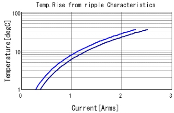
GRT033D70J105ME13 Temp. rise ■ 500kHz ■ 1MHz
