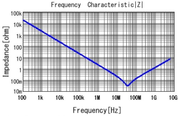
■ GRT033C80J104KE01 |Z| DCOV, 25degC
