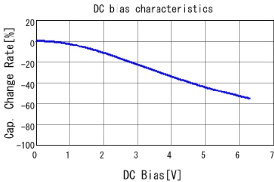
■ GRT033C70J104KE01 C-DC bias capchange, 25.0degC, AC0.
