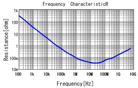
■ GRT033C70J104KE01 R DC0V, 25degC
