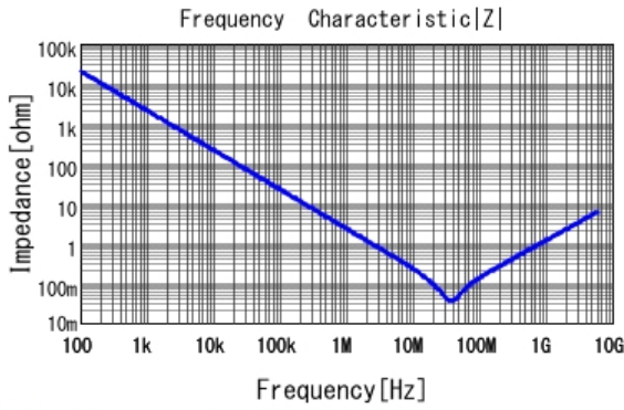
■ GRT033C70J104KE01 |Z| DC0V, 25degC
