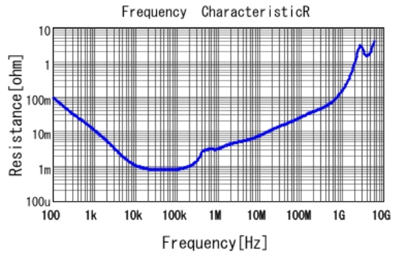
■ GRM32ER60E337ME05 R DCOV, 25degC
