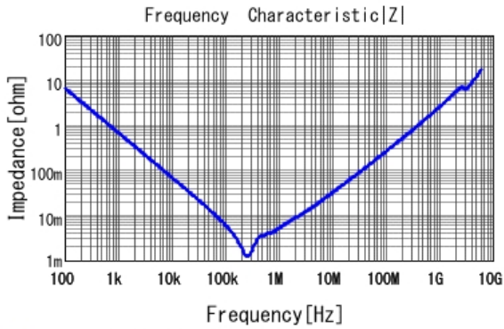
■ GRM32ER60E337ME05 |Z| DCOV, 25degC
