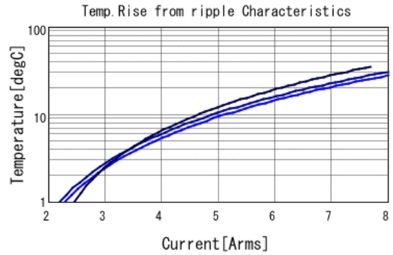
GRM32ER60E337ME05 Temp. rise ■ 50kHz ■ 200kHz ■ 400kHz
