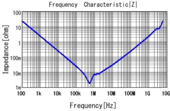
■ GRM32EE70J107ME15 |Z| DCOV, 25degC
