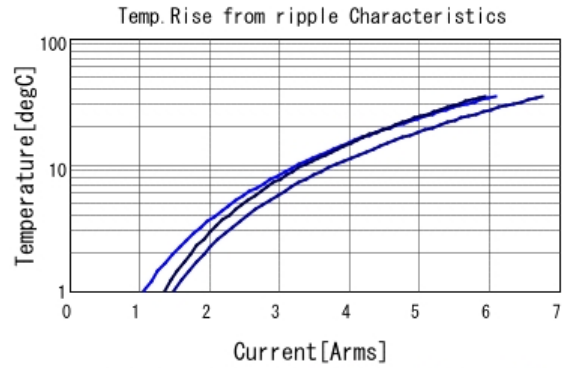
GRM32ED71A476KE15 Temp. rise ■ 60kHz ■ 300kHz ■ 600kHz
