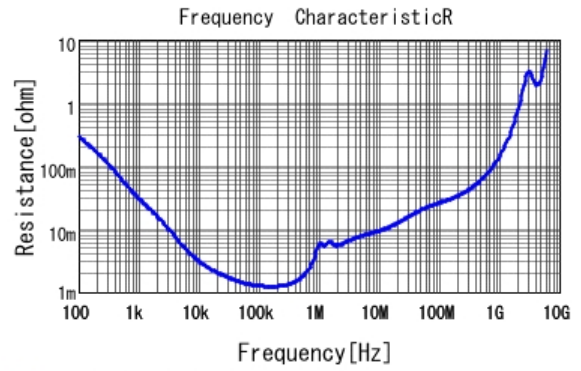
■ GRM32EC80J107ME20 R DCOV, 25degC
