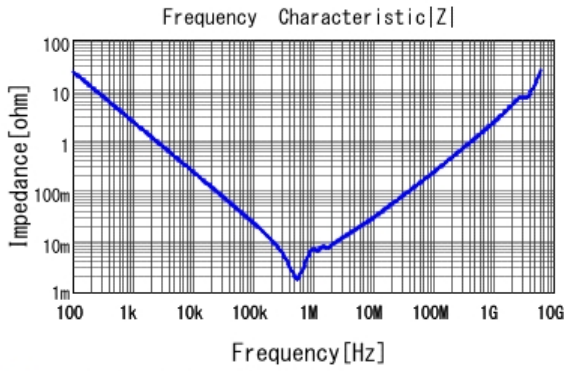
■ GRM32EC80J107ME20 |Z| DCOV, 25degC
