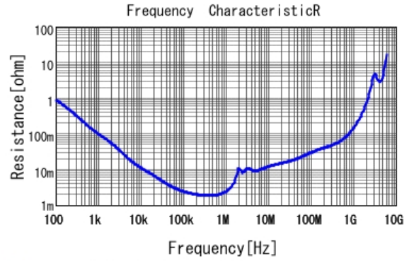
■ GRM32EB31E226ME15 R DCOV, 20degC
