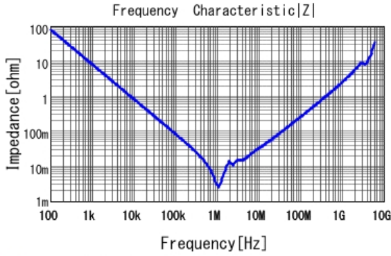
■ GRM32EB31E226ME15 |Z| DCOV, 20degC
