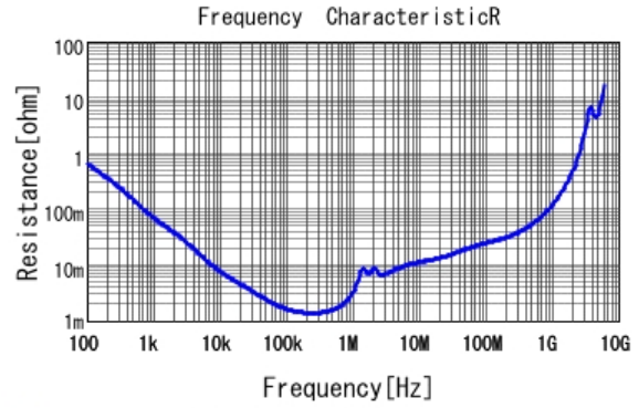
■ GRM32EB31C476KE15 R DCOV, 20degC
