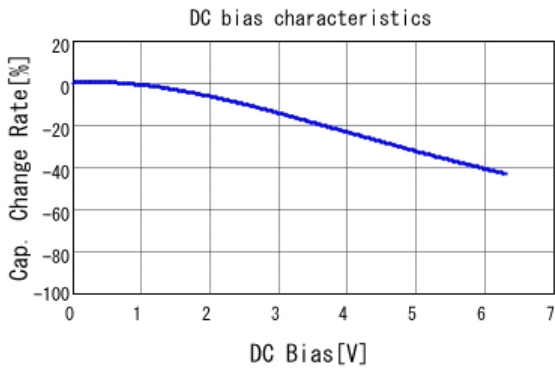
■ GRM32DR60J336ME19 C-DC bias capchange, 25.0degC, ACO.
