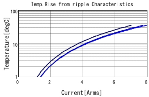
GRM31CC80E227ME11 Temp. rise ■ 50kHz ■ 200kHz ■ 400kHz
