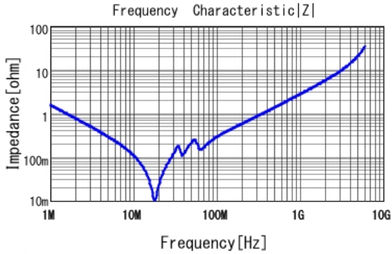
■ GRM3195C1H104GA05 |Z| DCOV, 25degC
