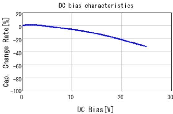
■ GRM21BR71E224KA01 C-DC bias capchange, 25.0degC, AC1.
