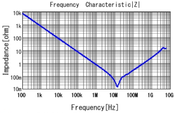
■ GRM21BR71E224KA01 |Z| DCOV, 25degC
