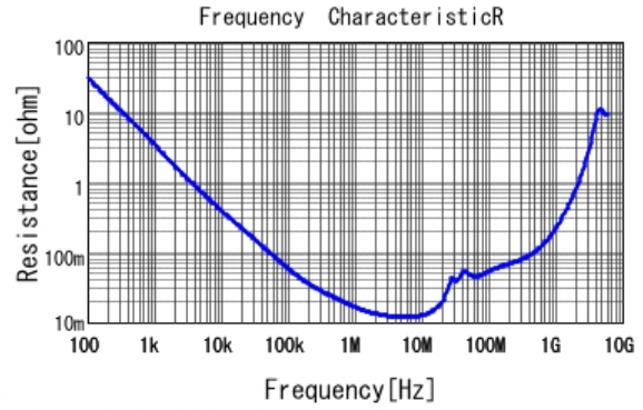
■ GRM21BR71E224KA01 R DCOV, 25degC
