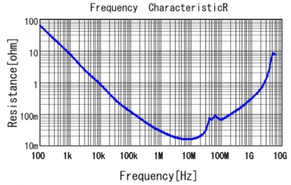
■ GRM21BR11H104KA01 R DCOV, 20degC
