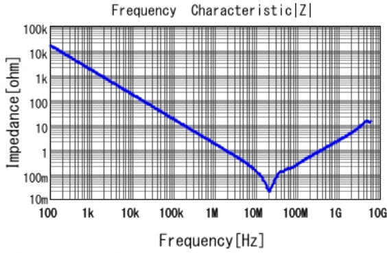
■ GRM21BR11H104KA01 |Z| DCOV, 20degC
